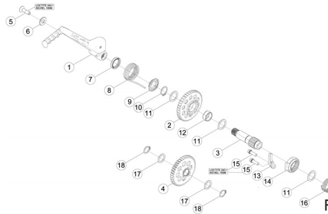
TAV.06 Avviamento a pedale - Kickstarter - Dé marriage à pedal - Pedalstart - Arranque a pedal
