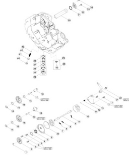
TAV.08 Impianto di lubrificazione - Lubrication system - Systê me de lubrification - Schmieranlage - Sistema de lubricaci3n
