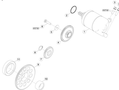
TAV.07 Avviamento elettrico - Electric starter - Dé marriage é lectrique - Elektrischer start - Arranque elé trico
